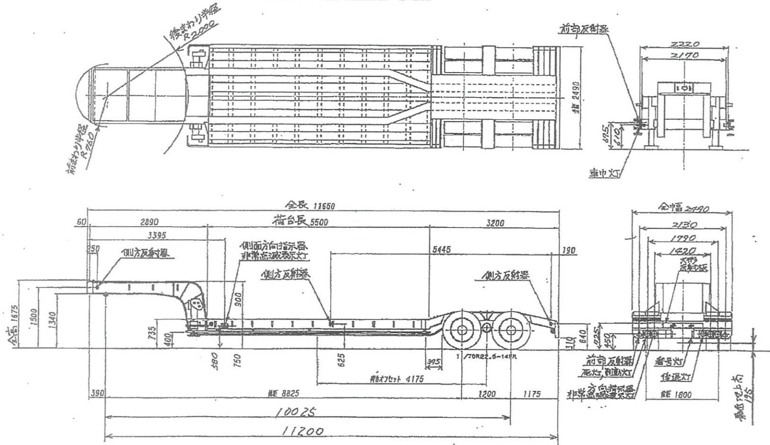
トレーラーモビル PMR238AA型 外形四面図
